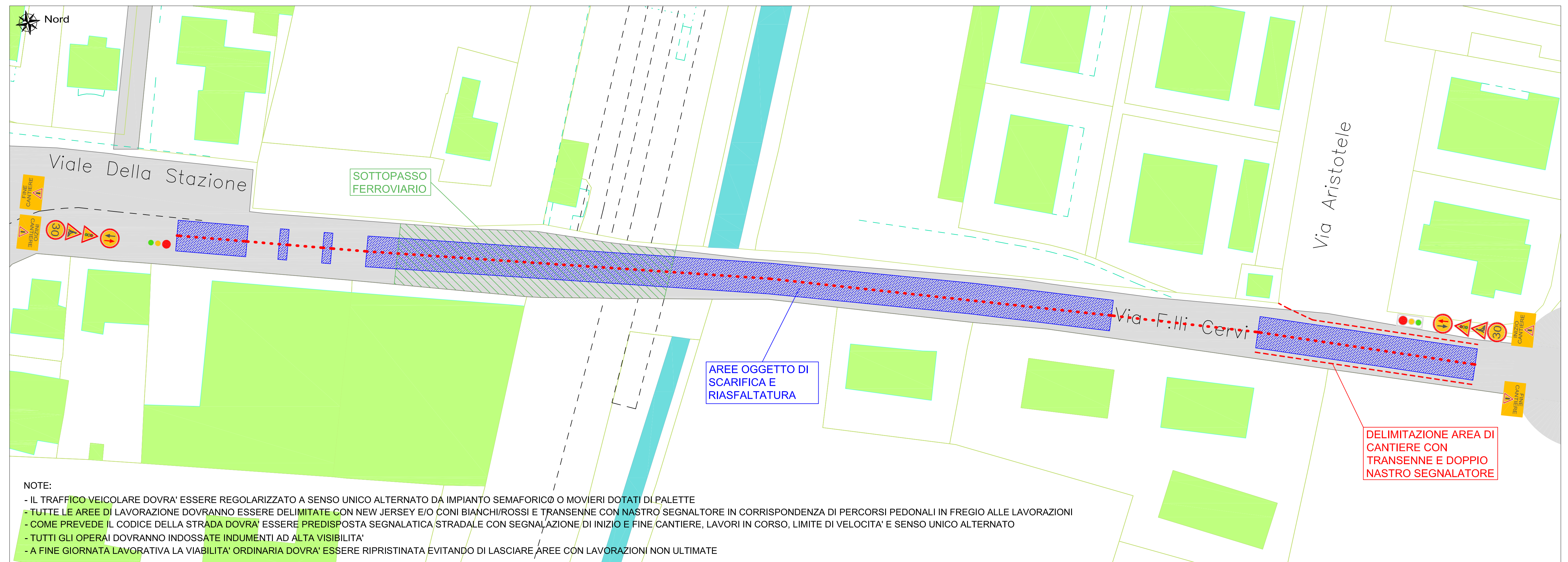
Via F.lli Cervi Layout di cantiere Scala 1:500
