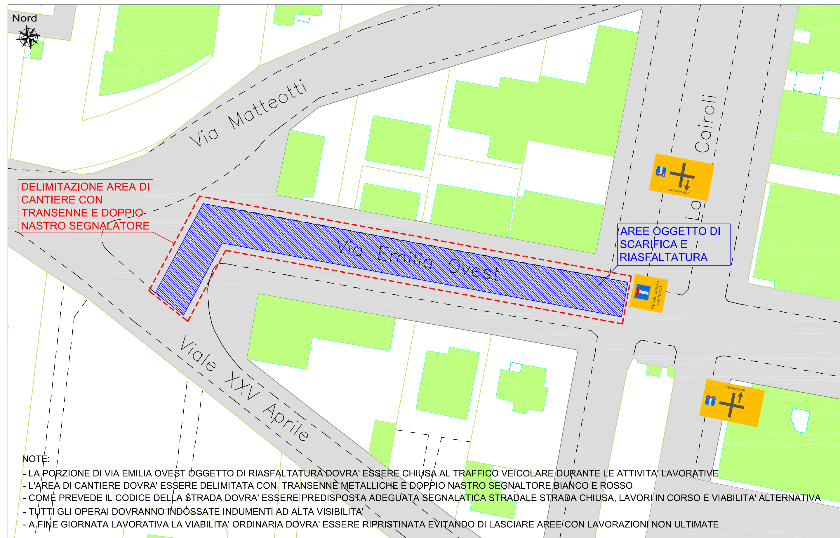
Via Emilia Ovest Layout di cantiere Scala 1:500
