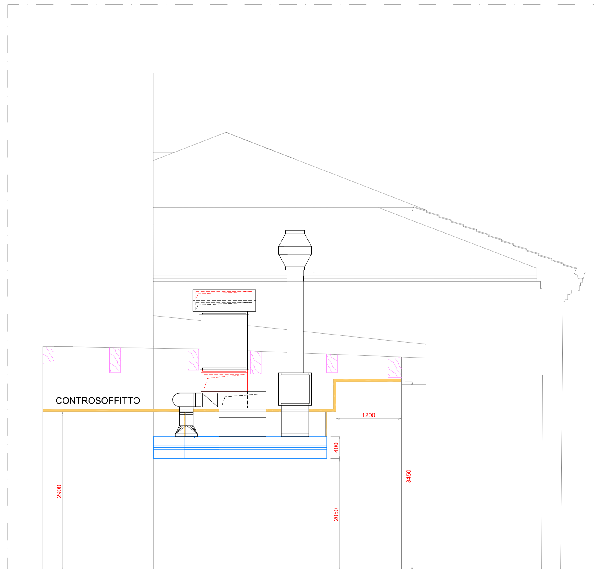
VISTA IN SEZIONE + (CONTROSOFFITTO)
