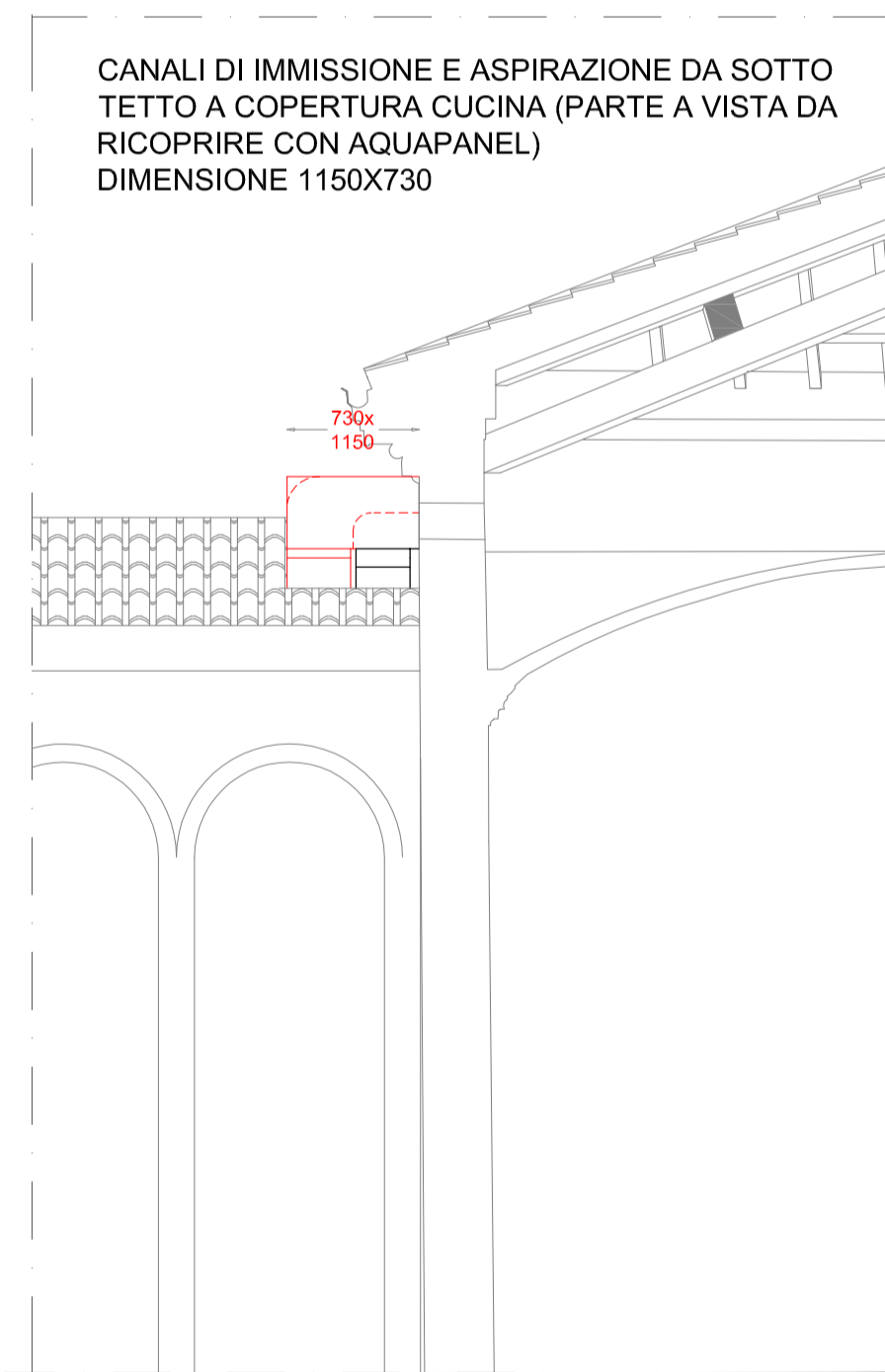
COPERTURA CANALI
