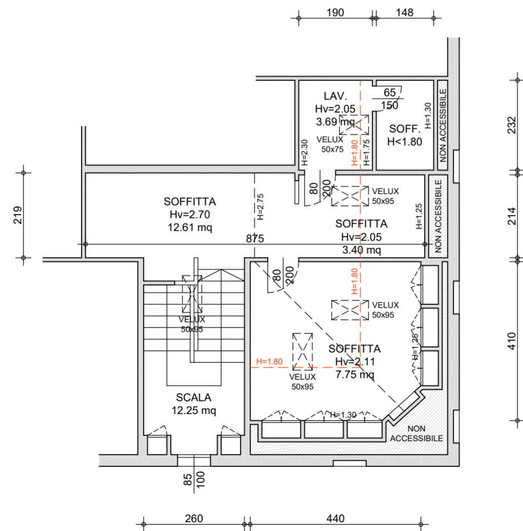
PIANTA PIANO SOTTOTETTO STATO DI FATTO
