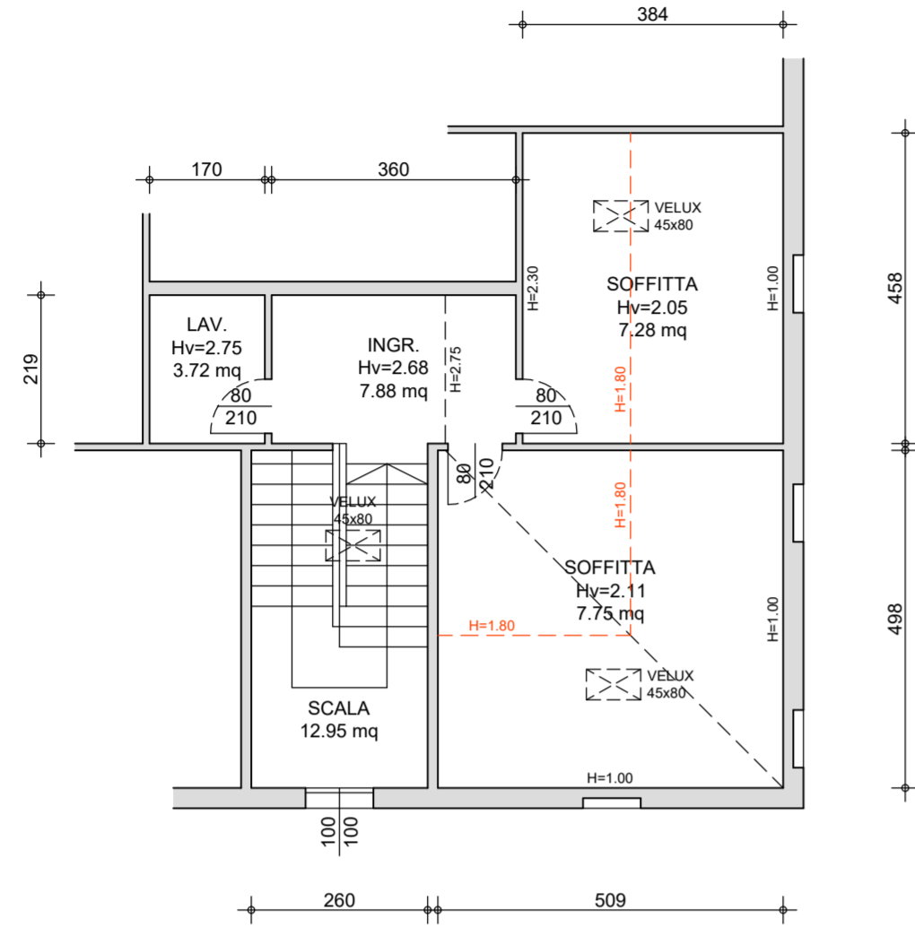
PIANTA PIANO SOTTOTETTO STATO LEGITTIMATO
