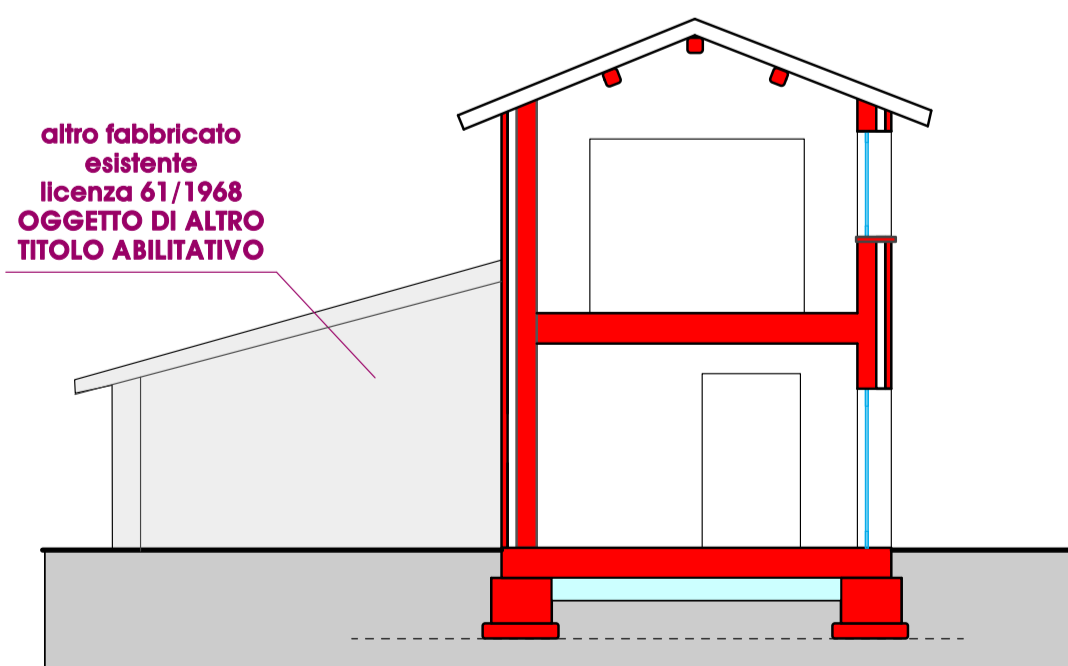
sezione AA
