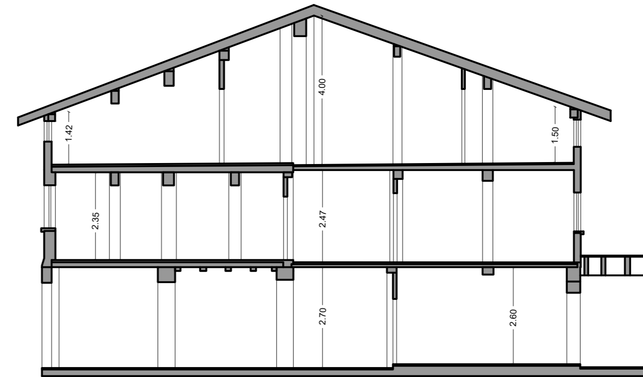
SEZIONE LONGITUDINALE
