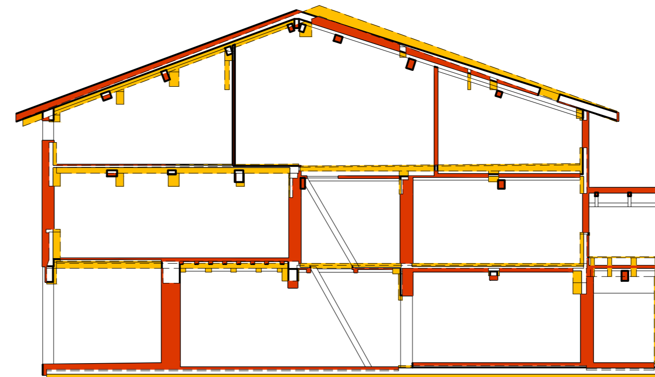
SEZIONE LONGITUDINALE
